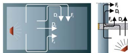
Schallübertragungswege
