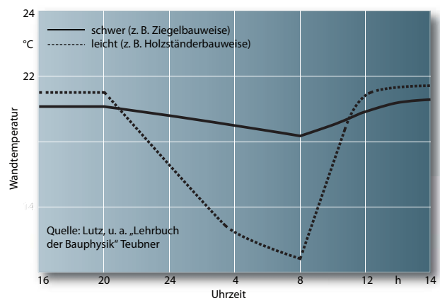
Auskühlverhalten eines Raumes
