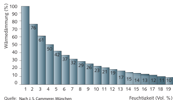
Abnahme des Dämmverhaltens von Mauerwerk bei zunehmender Durchfeuchtung
