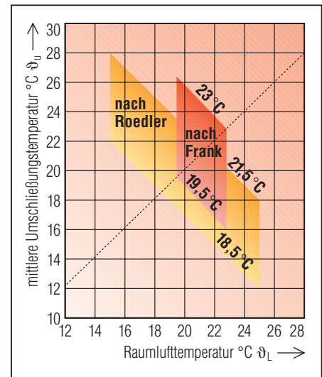
Bild 6 Behaglichkeitsfeld für das Wertepaar Raumlufttemperatur und Raumumschließungstemperatur.
