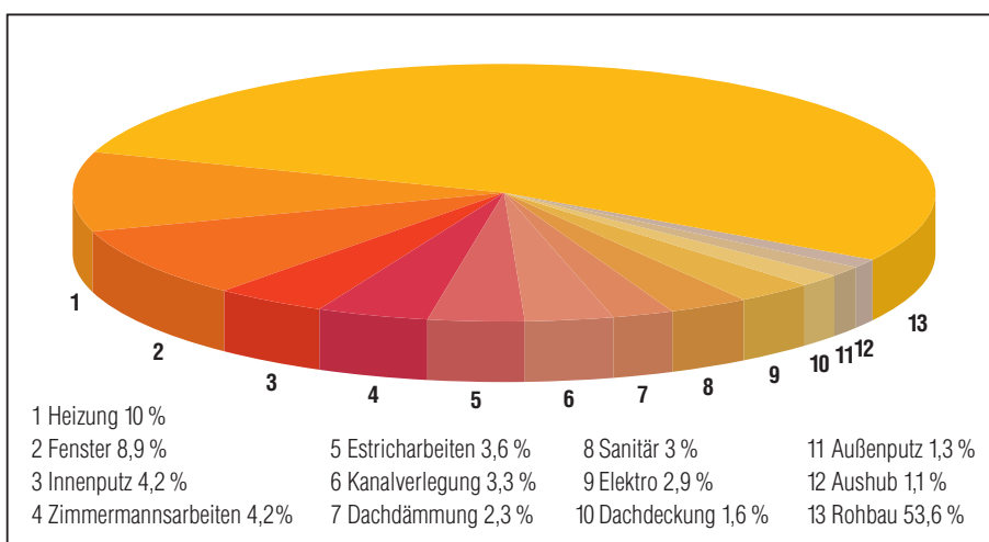
Bild 44 Anteile der untersuchten Gewerke am Primärenergiebedarf in den Lebensabschnitten „Errichtung und Instandhaltung“ [20] ohne Geräte und Ausbau.
