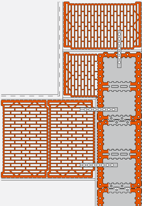
Abknickende Außenwand mit gefültem 42,5er UNIPOR Ziegel
