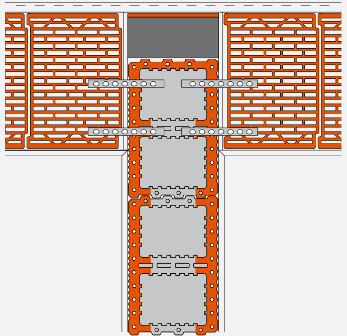
Außenwand mit 36,5er UNIPOR CORISO oder SILVACOR Ziegel
