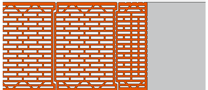
HALBER VERSTÄRKTER LAIBUNG SZIEGEL
