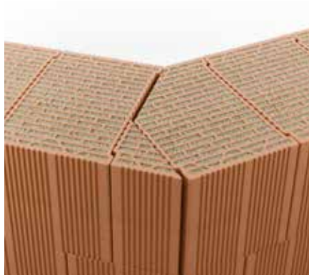
2. Mauerwerksschicht 36,5 cm
