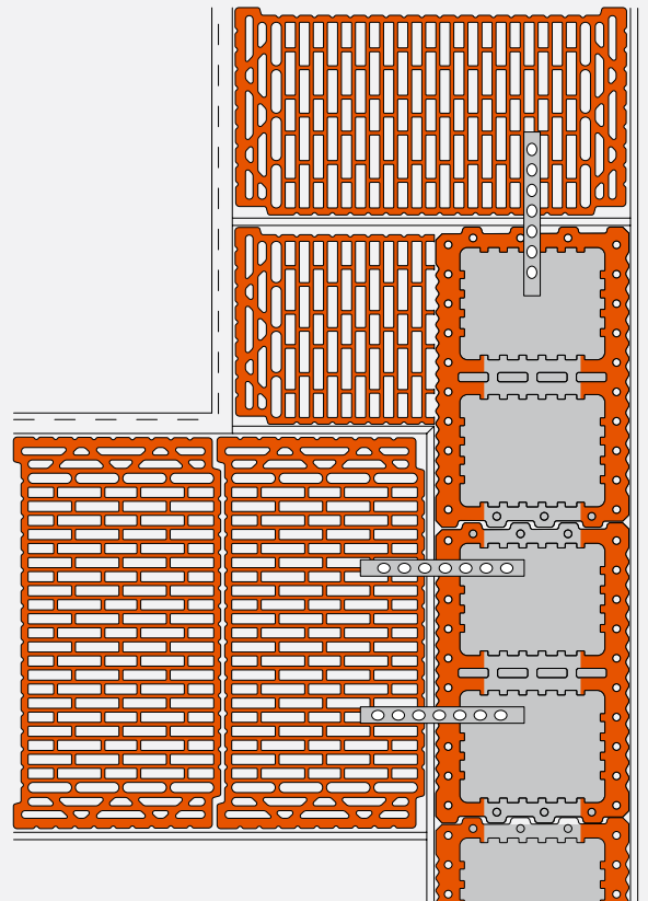
Abknickende Außenwand mit gefültem 49er UNIPOR Ziegel
