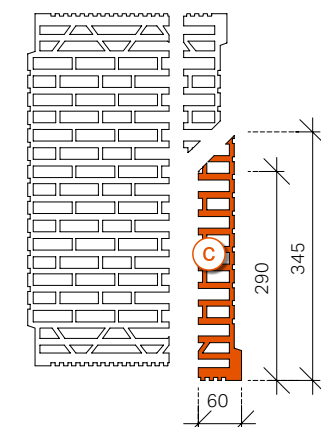
3. Scheibe absägen
