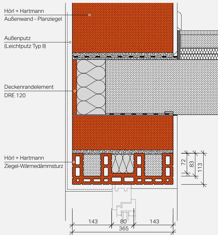
Einbindung eines Ziegel-Wärmedämmsturzes mit Höhenausgleichsziegel (HAZ) und Ziegel-Wärmedämmsturz
