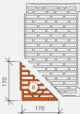
2. Ecke absägen
