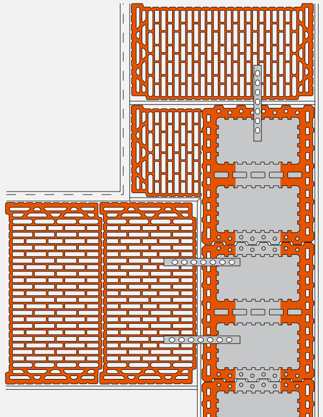
Abknickende Außenwand mit gefülltem 49er UNIPOR Ziegel
