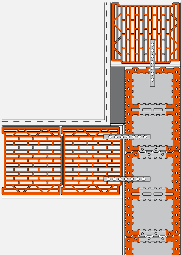
Abknickende Außenwand mit gefülltem 30er UNIPOR Ziegel
