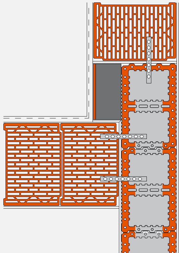
Abknickende Außenwand mit gefülltem 36,5er UNIPOR Ziegel
