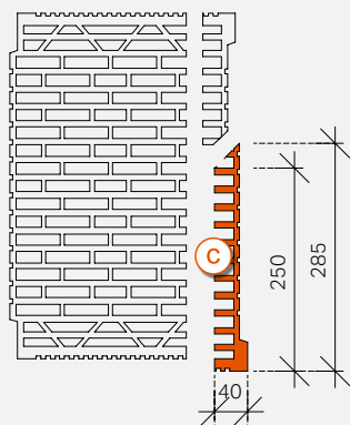
3. Scheibe absägen
